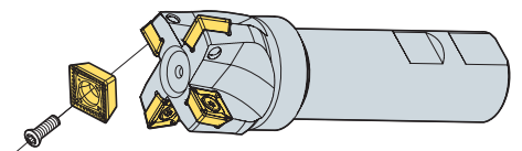
Схема сборки
