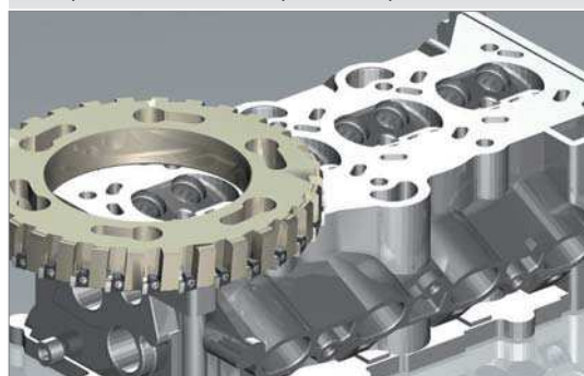
Черновая и чистовая обработка верхней плоскости
