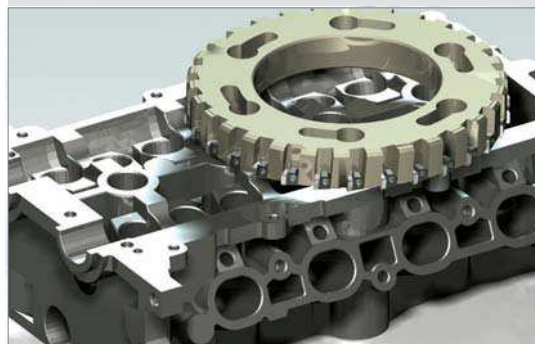
Черновая и чистовая обработка нижней плоскости
