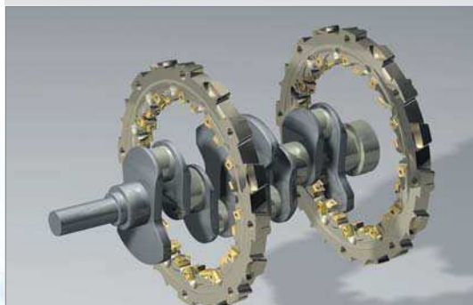
Внутреннее и внешнее фрезерование шеек коленчатого вала
